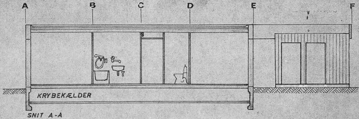
SNIT A-A
