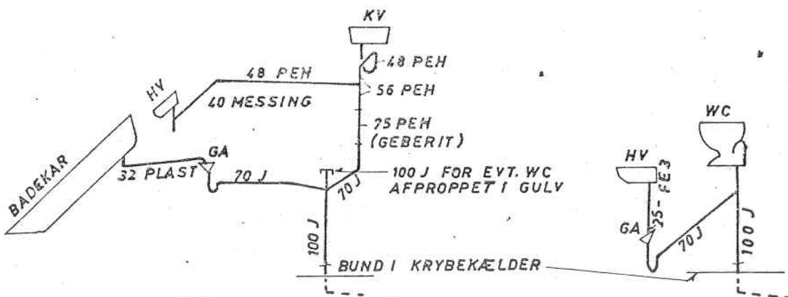
AFLØB FRA BAD OG KØKKENYASK
