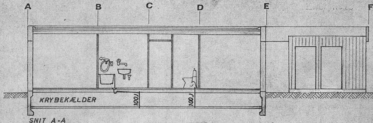
SNIT A-A
