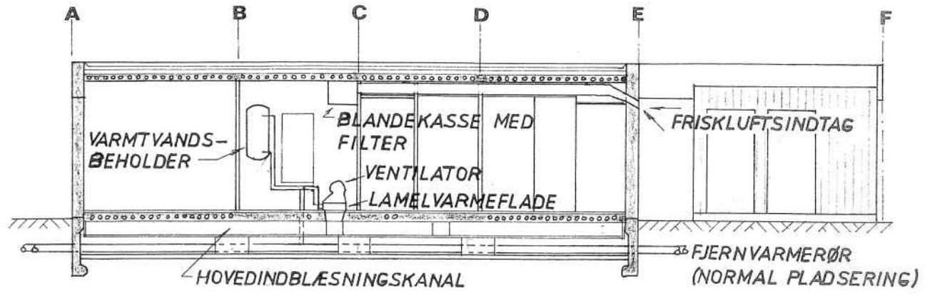
SNIT A-A
