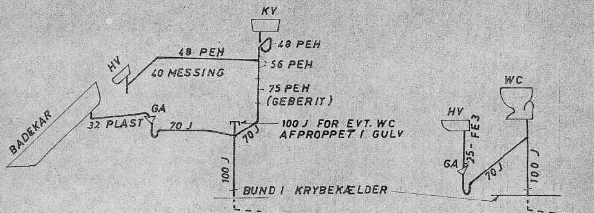
AFLØB FRA BAD OG KØKKENVASK
